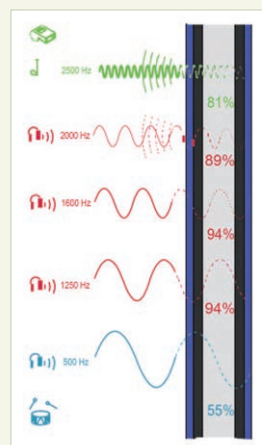
Absorptie waarde bij verschillende geluidsniveaus.
